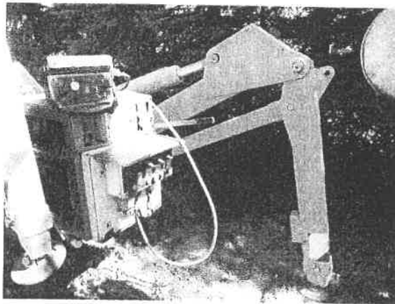
Zdj. nr 6. Zwyzka – pulpit sterowniczy maszyny oraz stabilizator
